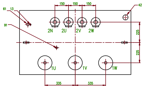
Pohled na víko
