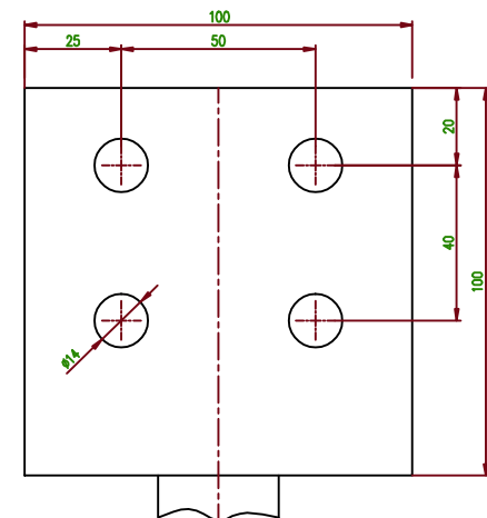
Připojovací kus FP M42
