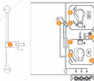
Ovl. mechanismus CI2 pojistkového odpínače a uzemňovače
