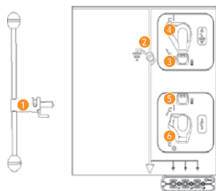
Ovládací mechanismy CI1 odpínače, CS1 odpojovače a CST uzemňovače
