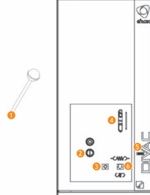
Ovládací mechanismus CDV vypínače Divac
